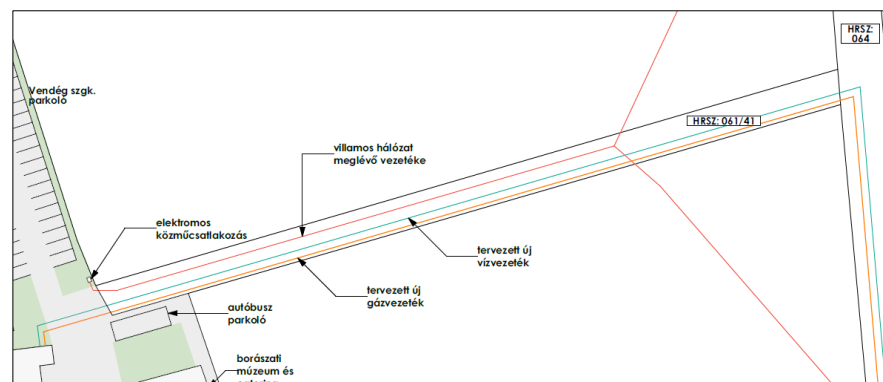
Tervezett új közművezetékek helye és a várható csatlakozási pont a telken belül
